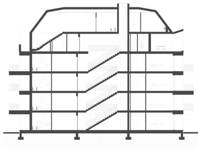
SECȚIUNE LONGITUDINALĂ
