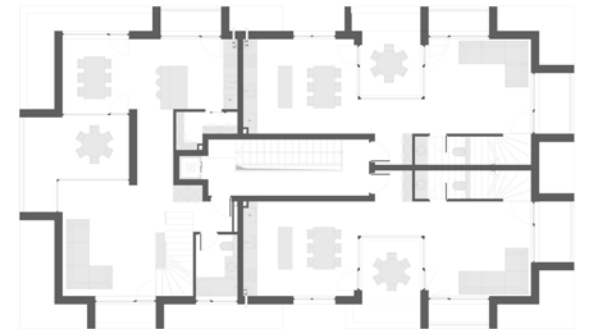
PLAN ETAJ RETRAS
